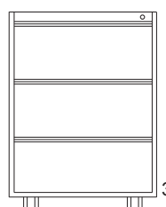
Vrhnji del iz jeklene pločevine pri R600
